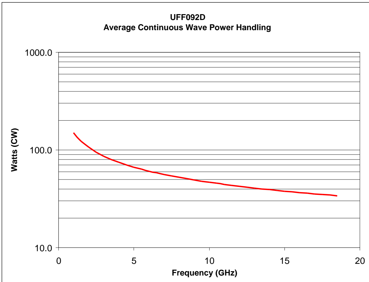
Fig. 8 UFF092D Power
