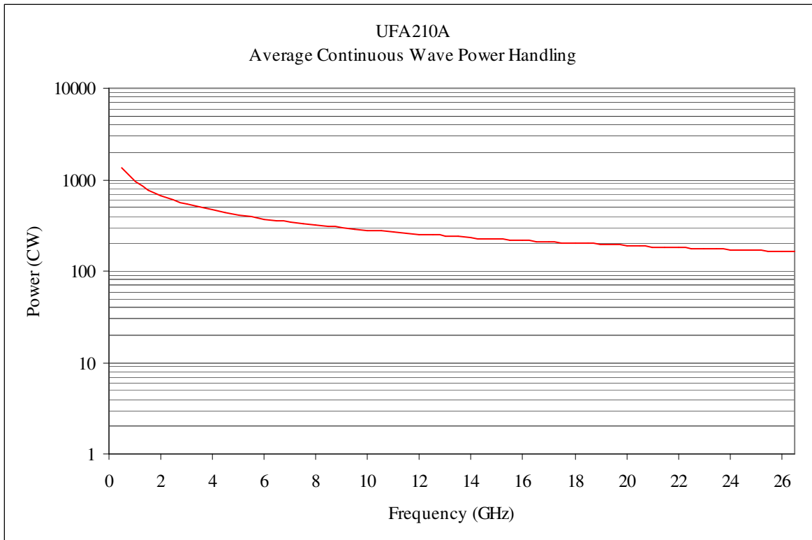
Fig. 8 UFA210A Power
