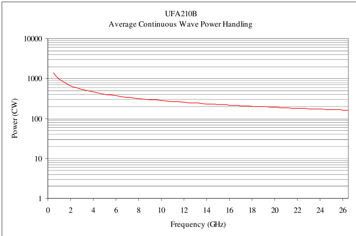
Fig. 8 UFA210B Power
