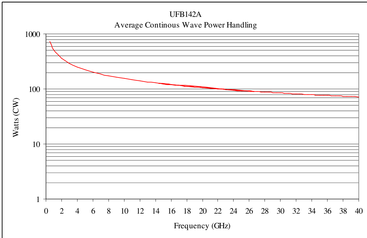
Fig. 8 UFB142A Power
