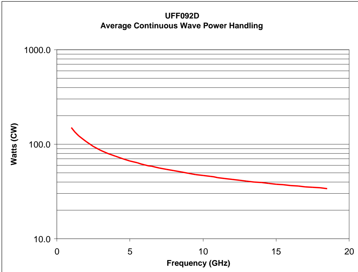
Fig. 8 UFF092D Power
